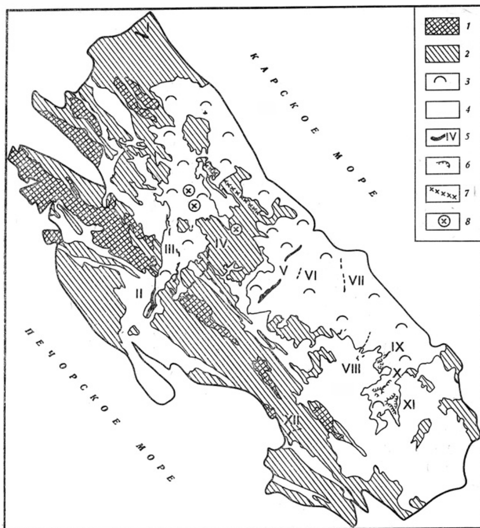
Геоморфологическая схема о. Вайгач.
